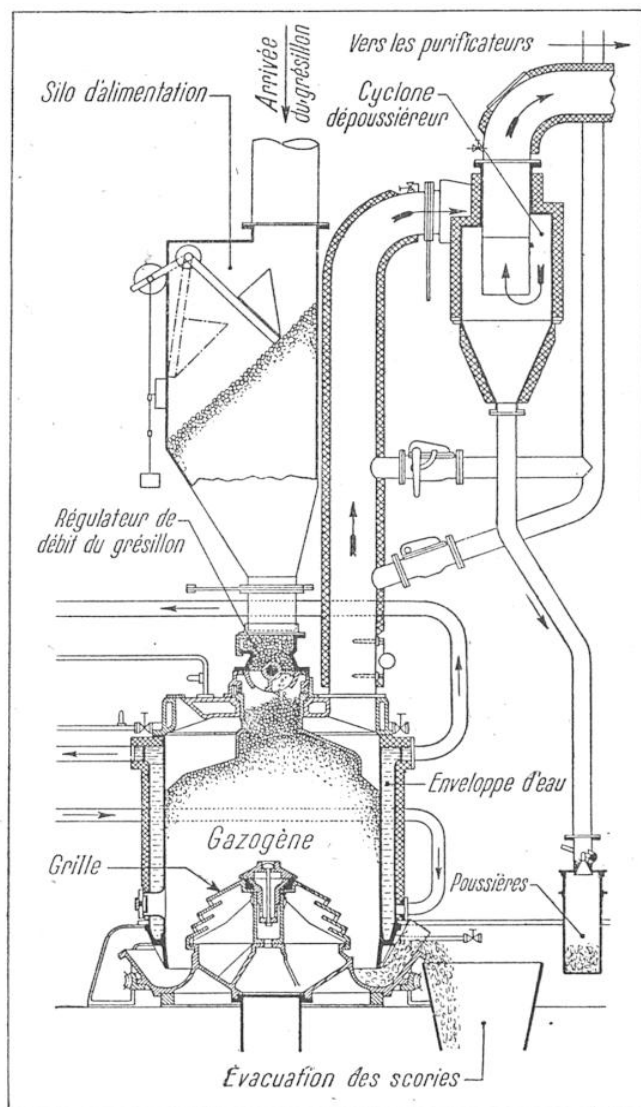
FIG. 4. — GAZOGÈNE A SILO BURMEISTER ET WAIN DU CARGO « NAVITAS »
