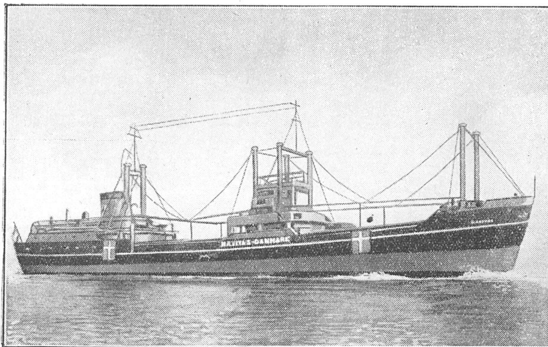
FIG. 3. — LE CARGO DANOIS « NAVITAS », PROPULSÉ PAR UN MOTEUR DIESEL FONCTIONNANT AU GAZ PAUVRE. Ce cargo, d'un port en lourd de 3 030 t, à deux cales, est propulsé par un moteur Diesel, Burmeister et Wain, transformé pour la marche au gaz de gazogène avec allumage électrique. Ce moteur à 6 cylindres développe, en service normal, une puissance de 950 ch à 140 tours/mn, la pression moyenne effective étant de 4,2 kg/cm 2 . Son équipement comporte en outre deux moteurs auxiliaires Diesel, transformés comme le précédent, de 100 ch chacun, et un moteur Diesel transformé en un véritable Diesel à gaz, de 50 ch. Ce dernier peut fonctionner, le cas échéant, soit au gas-oil, soit aux huiles de goudron de houille, sous-produits du fonctionnement des gazogènes.
