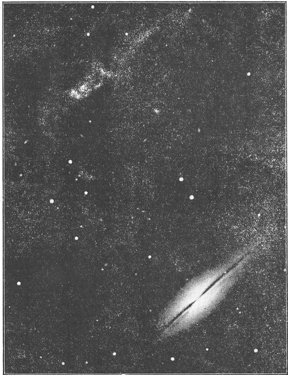
FIG. 7. — UN CHAMP DE PETITES NÉBULEUSES SPIRALES, PRÈS DE LA NÉBULEUSE H. II, 240, DANS LA CONSTELLATION DE PÉGASE
