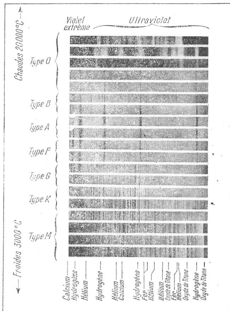
FIG. 4. — LES TYPES DE SPECTRES D'ÉTOILES
