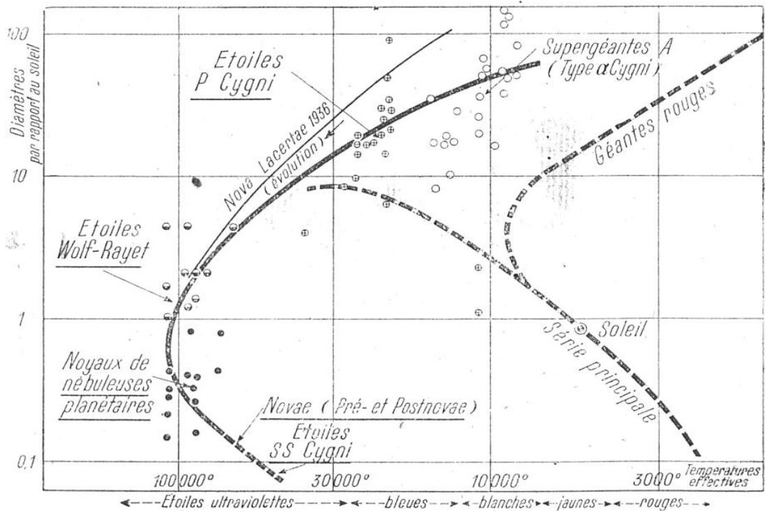
FIG. 6. — L'ÉVOLUTION DES NOVAE, ET LES ASTRES QUI LEUR SONT APPARENTÉS
