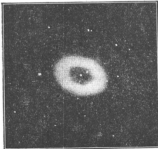
FIG. 3. — LA NÉBULEUSE ANNULAIRE DE LA LYRE PHOTOGRAPHIÉE À L'OBSERVATOIRE DU MONT WILSON
