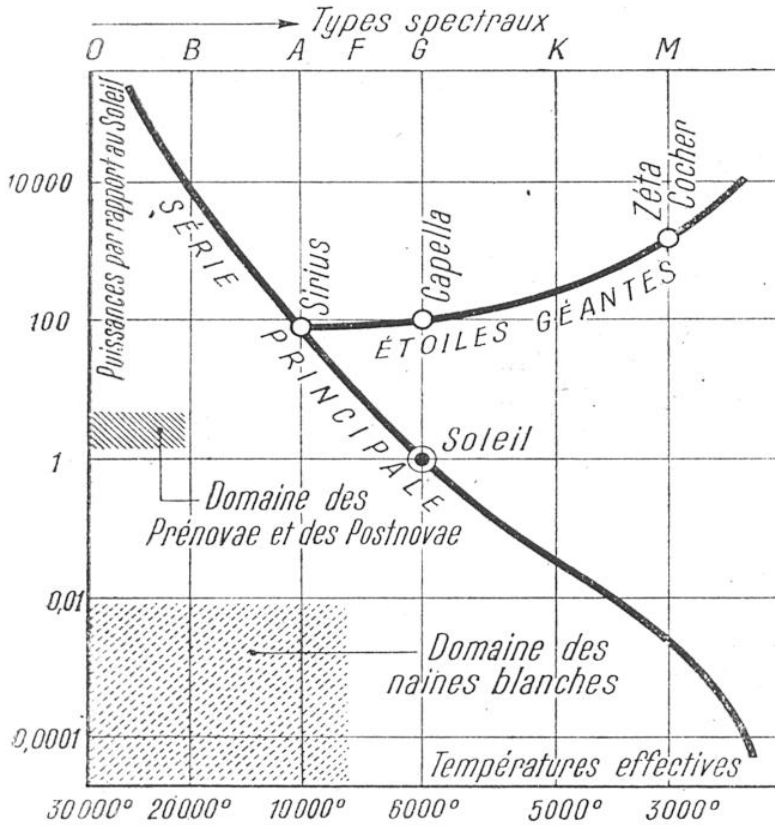
FIG. 2. — LE DIAGRAMME DE HERZSPRUNG-RUSSELL
