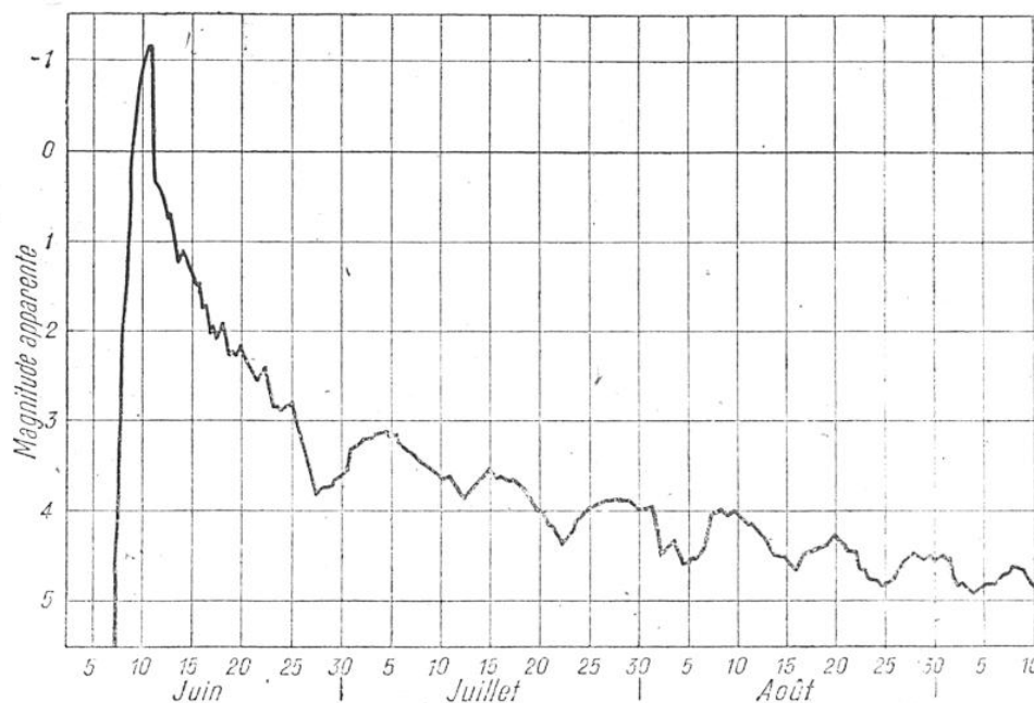
FIG. 1. — COURBE DE LUMIÈRE DE NOVA AQUILÆ 1918, PENDANT LES TROIS MOIS QUI SUIVIRENT SON APPARITION DANS LE CIEL
