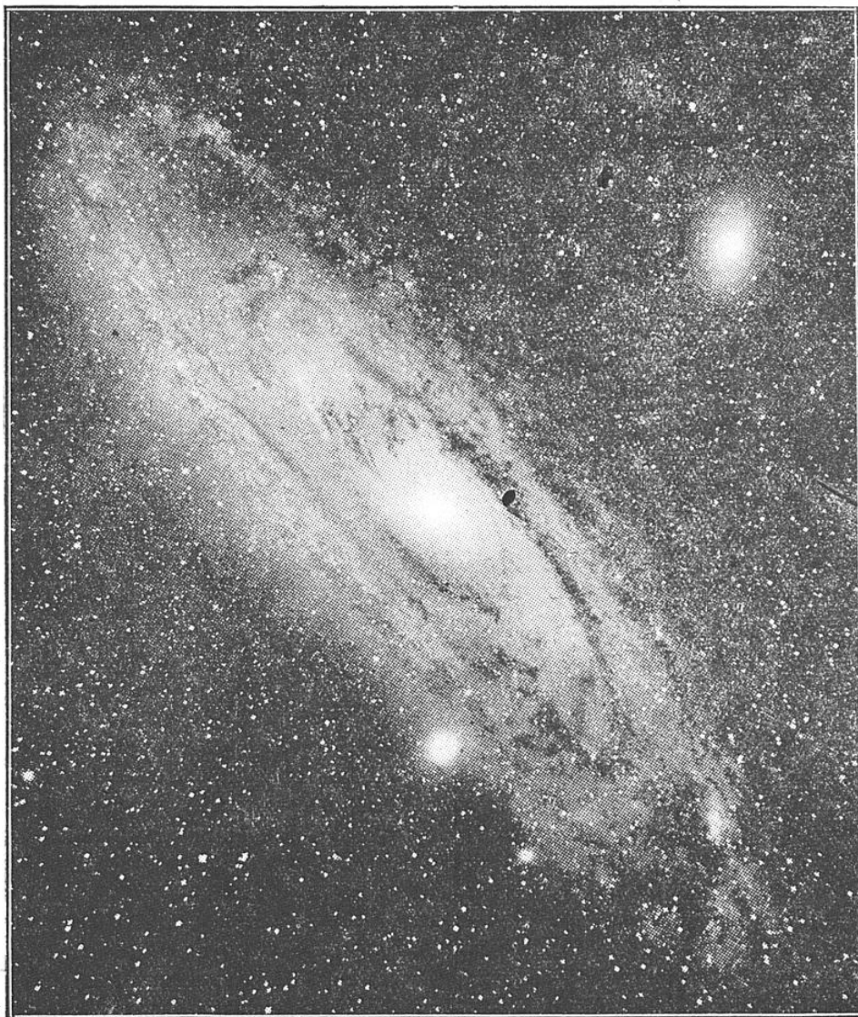
FIG. 5. — LA GRANDE NÉBULEUSE SPIRALE D'ANDROMÈDE (MESSIER 31)
