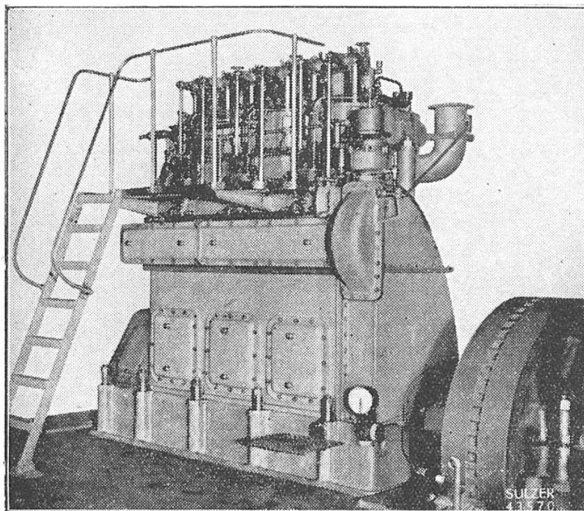
FIG. 1. — MOTEUR DIESEL À GAZ DE LA COMPAGNIE DE CONSTRUCTIONS MÉCANIQUES, PROCÉDÉS SULZER
