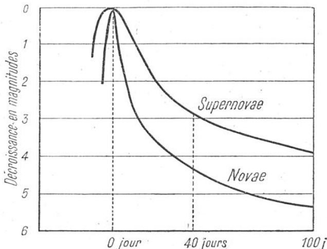
FIG. 8. — COMPARAISON DES COURBES DE LUMIÈRE MOYENNES DES NOVAE ET DES SUPERNOVAE
