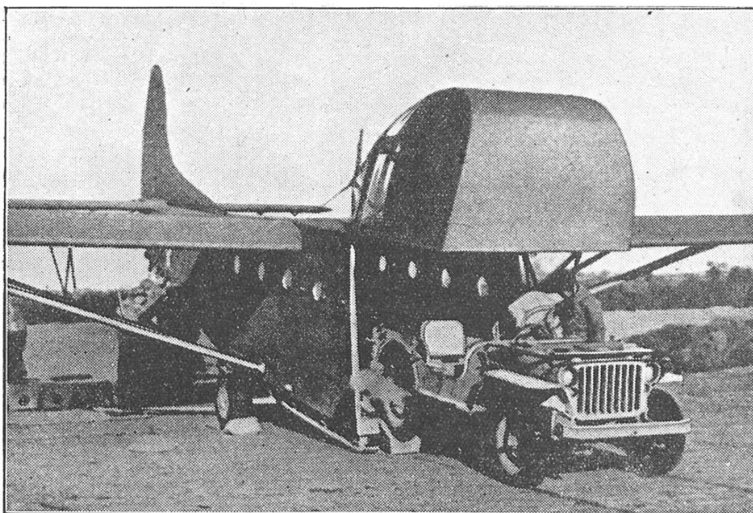
FIG. 5. — LE PLANEUR AMÉRICAIN WACO CG-4 CHARGEANT UNE VOITURETTE DE RECONNAISSANCE Tout l'avant du planeur est relevable pour donner rapidement passage au véhicule transporté.
