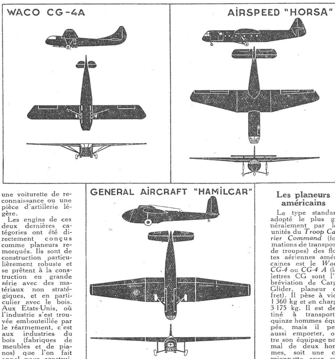
FIG. 1. — LES PLANEURS DE FRET ET DE TRANSPORT DES TROUPES ALLIÉS DU DÉBARQUEMENT AÉRIEN DE NORMANDIE
