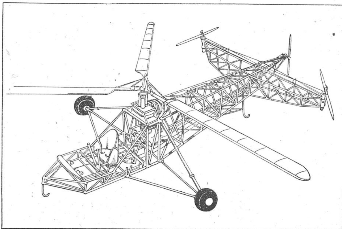
FIG. 1. — LE PREMIER HÉLICOPTÈRE VOGHT-SIKORSKY DE 1940
