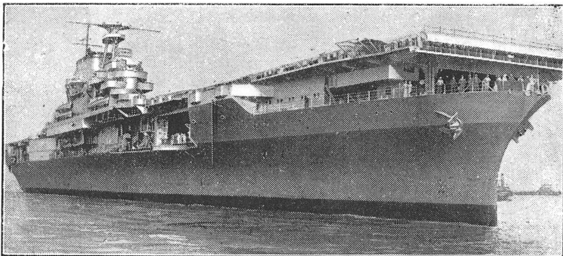
FIG. 1. — LE « HORNET », PORTE-AVIONS DE LA MARINE AMÉRICAINE, MIS EN SERVICE FIN OCTOBRE 1941 ET PERDU UN AN PLUS TARD DANS LES BATAILLES DES ILES SALOMON
