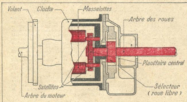
FIG. 8. — SCHÉMA DE LA TRANSMISSION A INERTIE HOBBS
