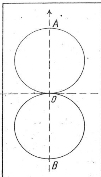
FIG. 1. — DIAGRAMME DE RAYONNEMENT D'UN CADRE COMPENSÉ
