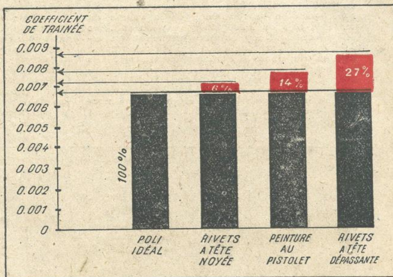
FIG. 11. — INFLUENCE DU POLI DE LA SURFACE SUR LA TRAINÉE DE FROTTEMENT
