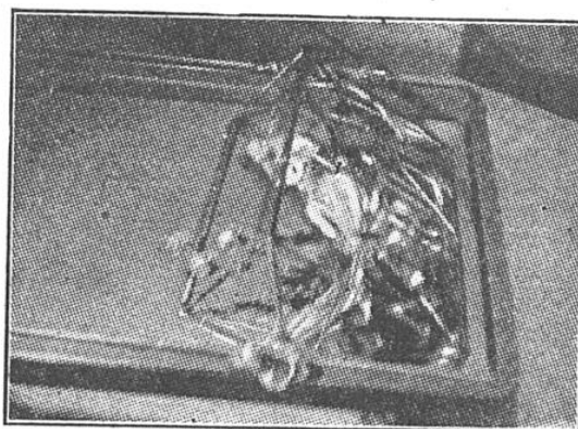
FIG. 2. — LE SIÈGE DU PILOTE, SUSPENDU À L'EXTREMITÉ DU BRAS MOBILE, S'INCLINE SOUS L'EFFET DE LA FORCE CENTRIFUGE
