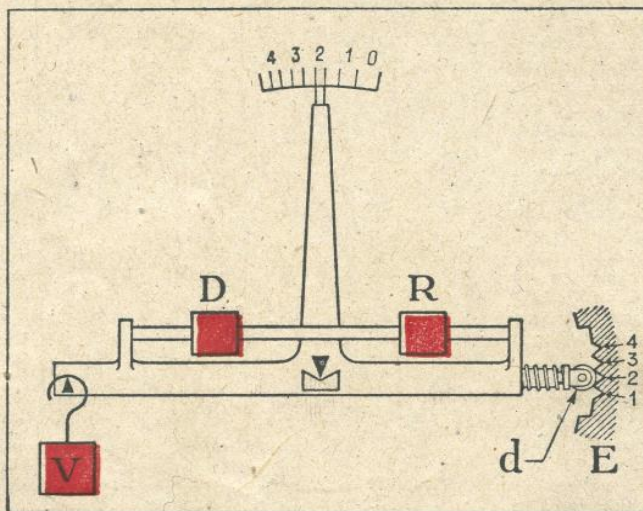
FIG. 3. — RÉALISATION DE PRINCIPE D'UN DÉCLENCHÉUR DE CHANGEMENT DE VITESSE AUTOMATIQUE
