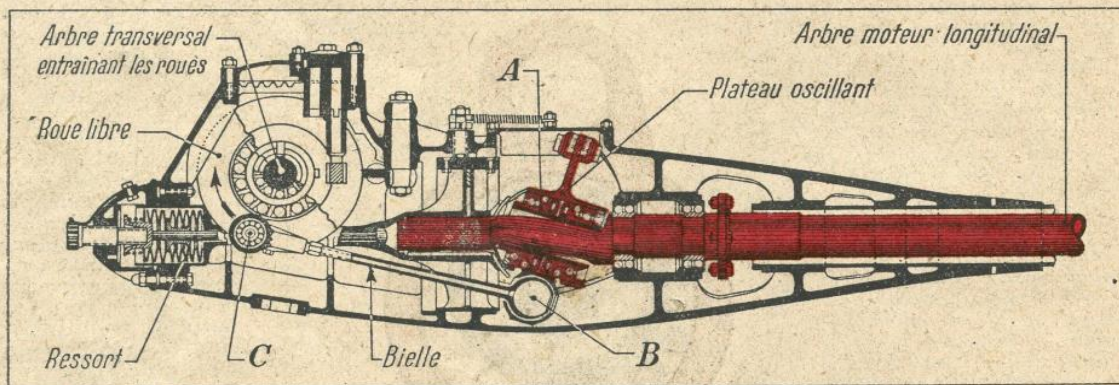
FIG. 5. — CHANGEMENT DE VITESSE AUTOMATIQUE SENSAUD DE LAVAUD A PLATEAU OSCILLANT
