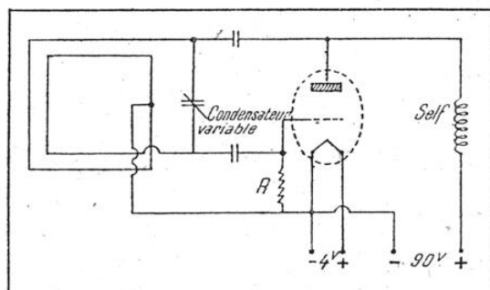
FIG. 2. — PRINCIPE DE L'OSCILLATEUR A CADRE COMPENSÉ
