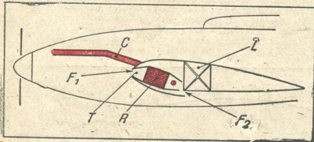
FIG. 5. — MONTAGE ROLLS-ROYCE D'UN RADIATEUR DANS L'AILE
