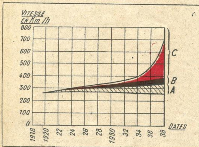
FIG. 1. — GRAPHIQUE MONTRANT L'INFLUENCE RESPECTIVE DE L'ACCROISSEMENT DE LA PUISSANCE (ZONE A) DE L'ADOPTION DE COMPRESSION (ZONE B) ET DE L'AMÉLIORATION DE LA FINESSE (ZONE C) SUR LA VITESSE DES AVIONS
