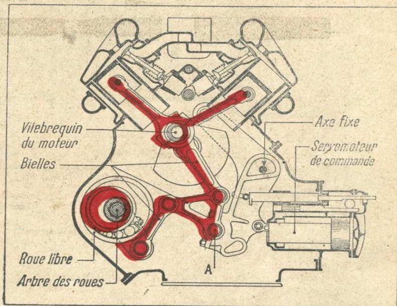
FIG. 6. — LE CHANGEMENT DE VITESSE MÉCANIQUE CONTINU R v R
