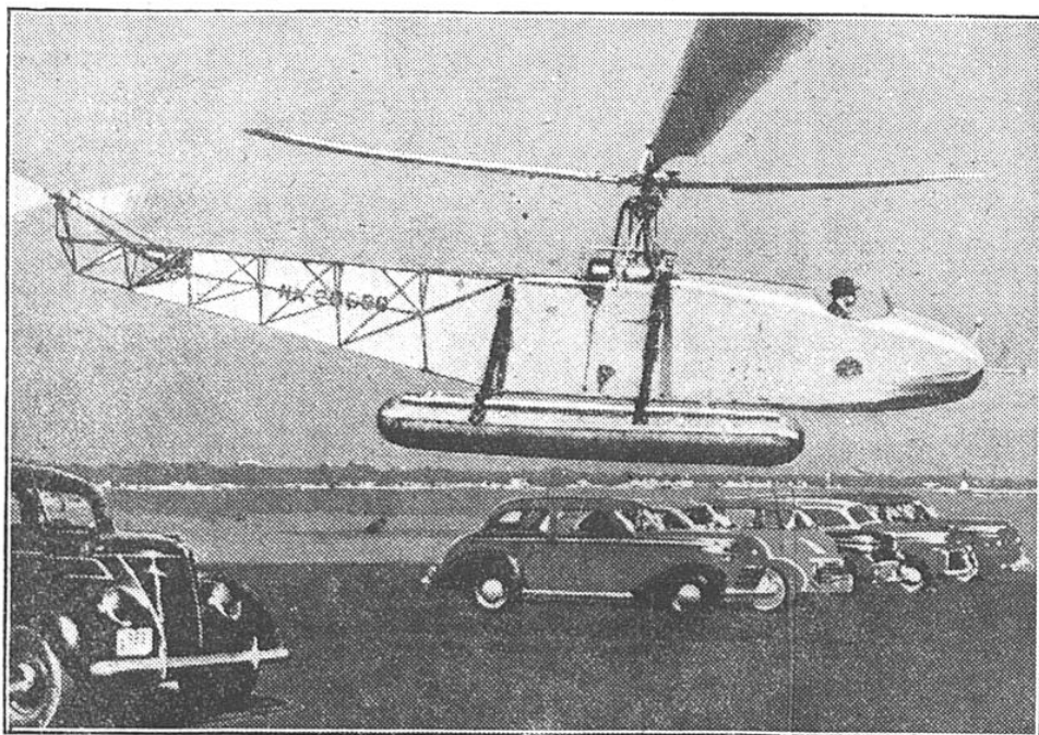
FIG. 3. — L'HÉLICOPTÈRE V S-300 A, TYPE 1943, EFFECTUANT UN ATTERRISSAGE DE PRÉCISION
