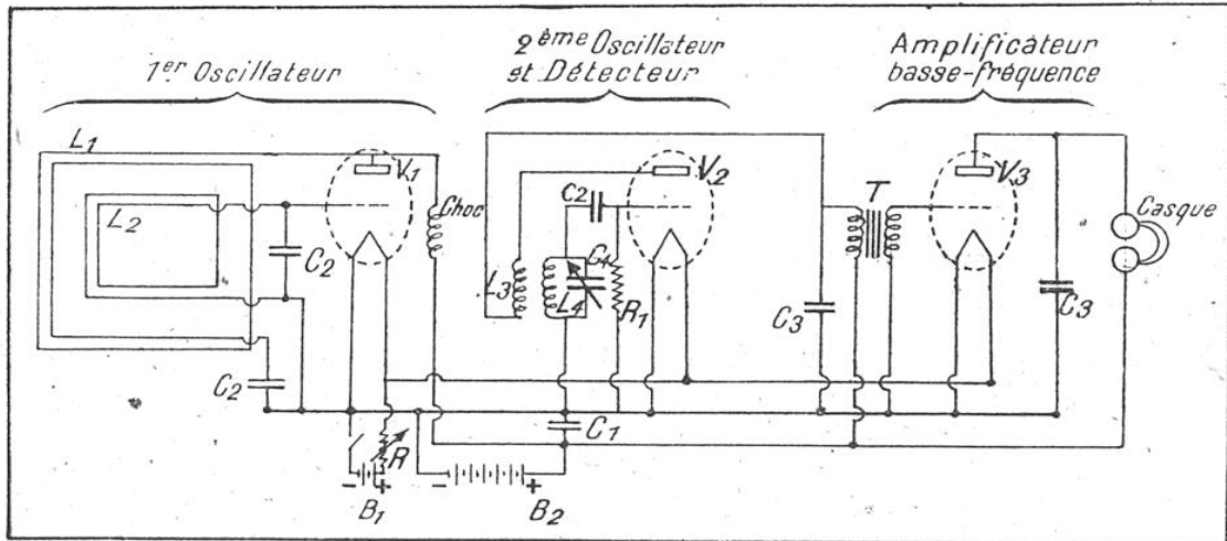
FIG. 3. — SCHÉMA D'UN DÉTECTEUR ÉLECTROMAGNÉTIQUE A CADRE UNIQUE
