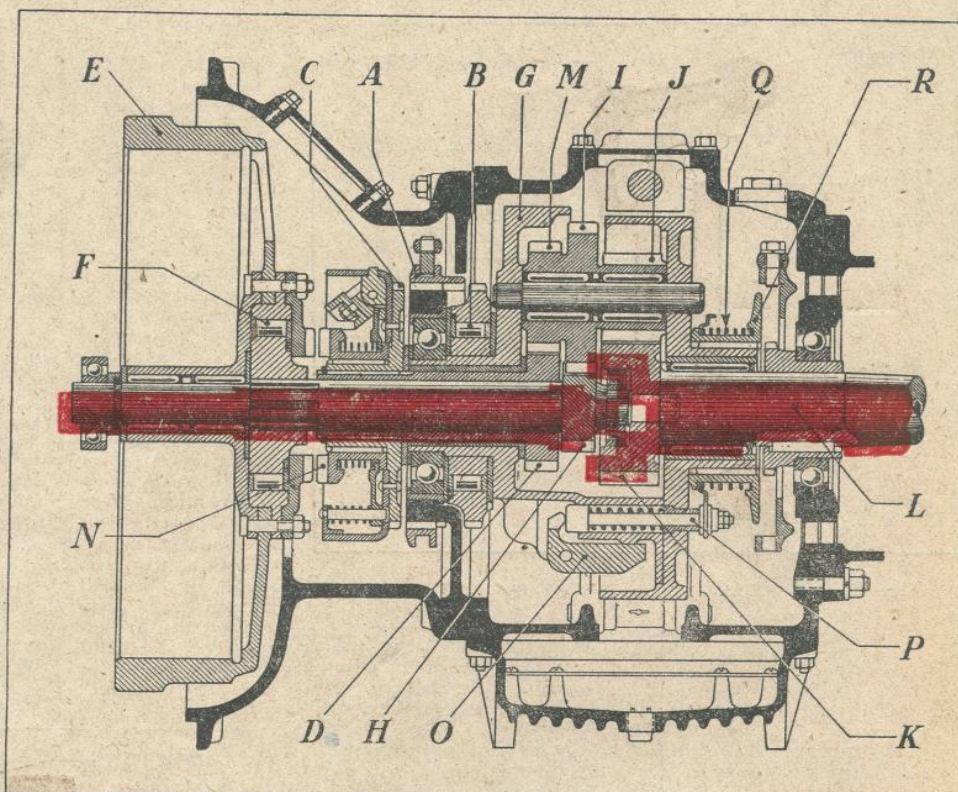
FIG. 12. — COUPE LONGITUDINALE DU CHANGEMENT DE VITESSE AUTOMATIQUE A BALADEUR DE LA YELLOW COACH
