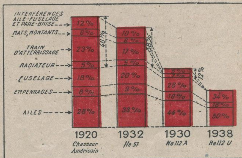
FIG. 2. — GRAPHIQUE MONTRANT L'ÉLIMINATION PROGRESSIVE DES RÉSISTANCES PARASITES
