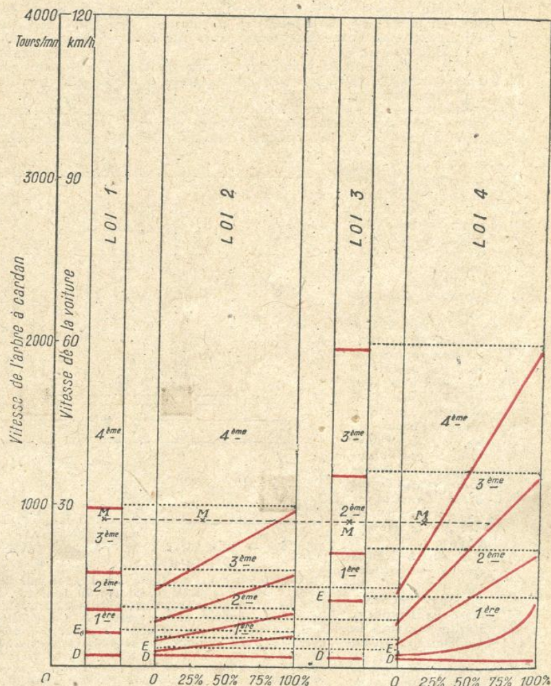
FIG. 2. — LES LOIS DE CONDUITE D'UNE VOITURE AUTOMOBILE
