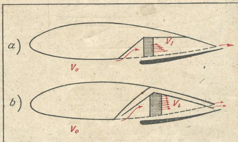
FIG. 4. — MONTAGES DU RADIATEUR DANS L'AILE EN VUE DE RÉDUIRE LA RÉSISTANCE EXTÉRIEURE DE CET ORGANE
