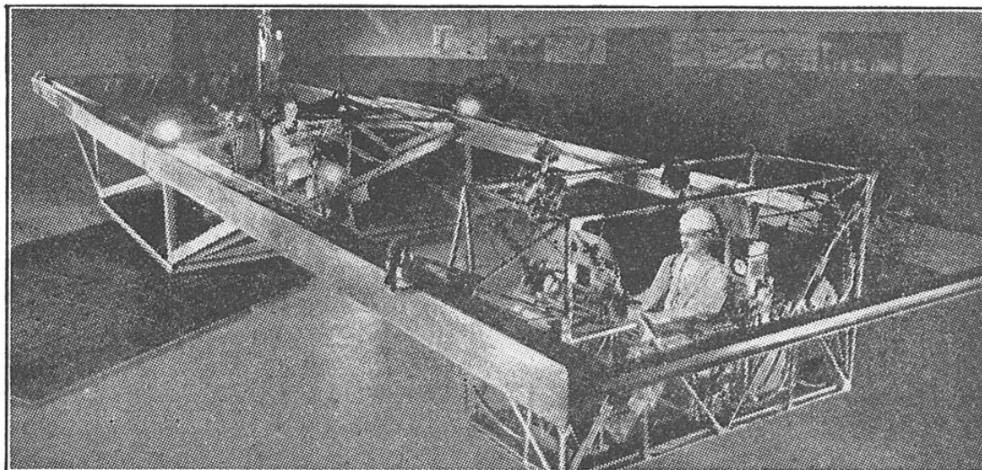
FIG. 1. — LE CARROUSEL DE WRIGHT FIELD POUR L'ÉTUDE DU « MAL DES ACCÉLÉRATIONS »
