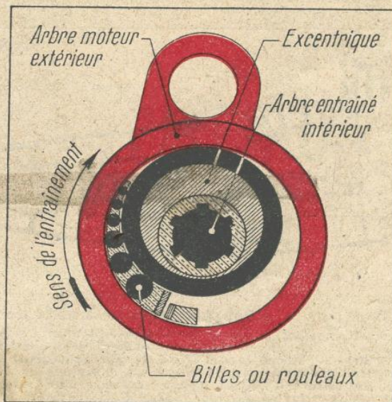
FIG. 4. — LE DISPOSITIF DE ROUE LIBRE R. V. R. (ROBIN VAN ROGGEN)
