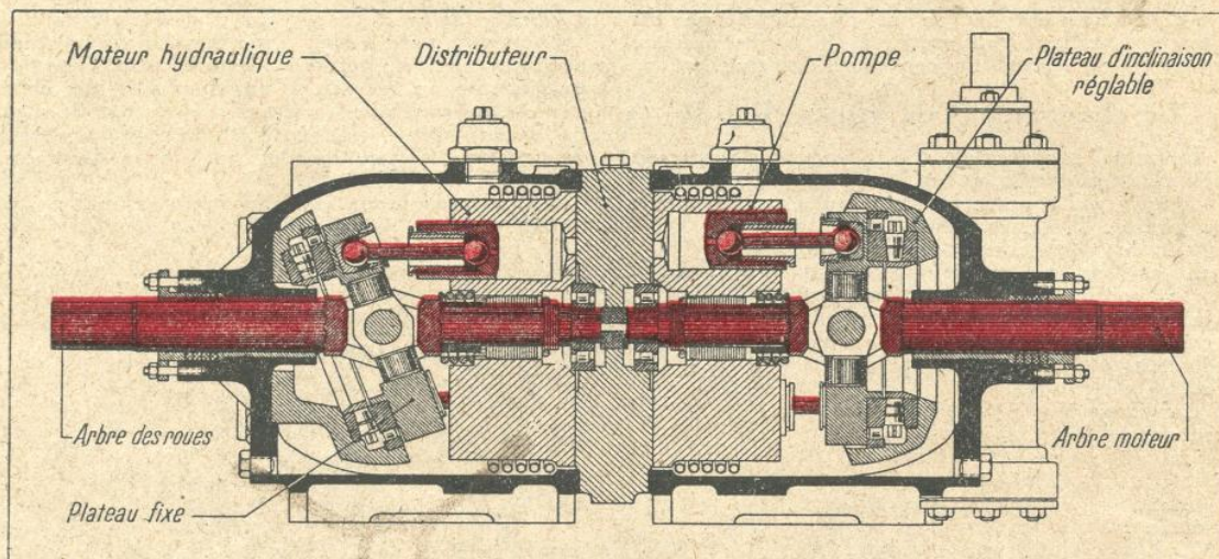
FIG. 7. — LE CONVERTISSEUR DE COUPLE HYDRAULIQUE WATERBURY
