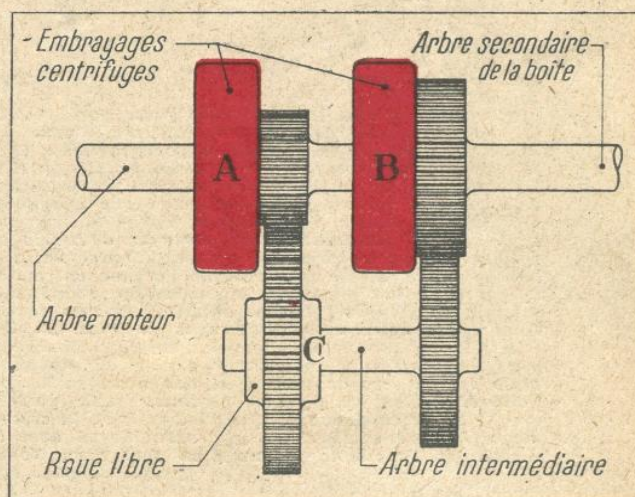
FIG. 11. — SCHÉMA D'UN CHANGEMENT DE VITESSE À DEUX VITESSES, COMPLÈTEMENT AUTOMATIQUE (STURTEVANT)
