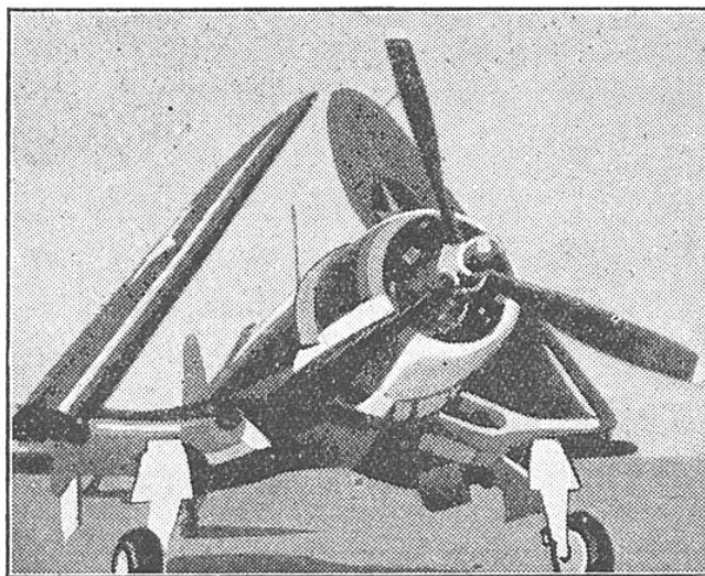
FIG. 8. — LE CHASSEUR VOGHT-SIKORSKY « CORSAIR » POSSÈDE DES DEMI-AILES RELEVABLES POUR DIMINUER SON ENCOMBREMENT DANS LES HANGARS DES PORTE-AVIONS SUR LESQUELS IL EST EMBARQUÉ
