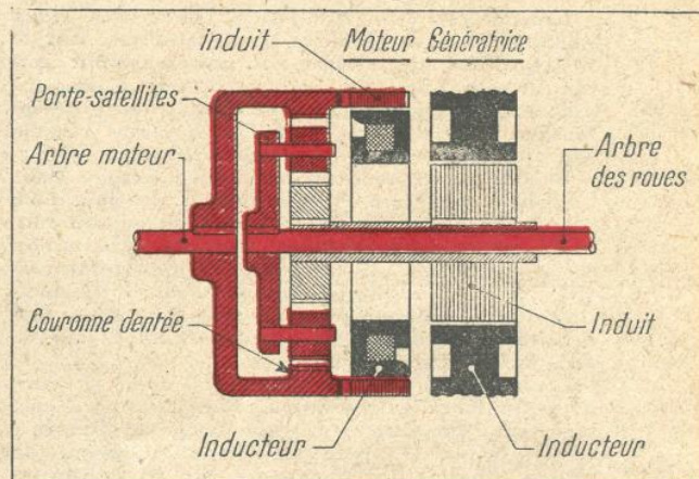
FIG. 14. — SCHÉMA D'UN CHANGEMENT DE VITESSE DIFFÉRENTIEL ÉLECTRIQUE CONTINU
