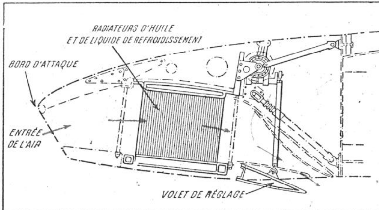
FIG. 8. — COUPE DU RADIATEUR DU DESTROYER BIMOTEUR DE HAVILLAND « MOSQUITO »
