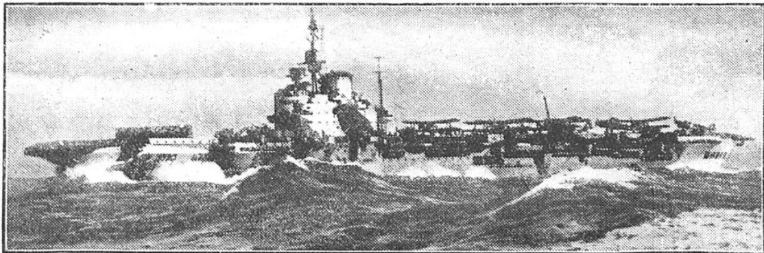
FIG. 2. — LE PORTE-AVIONS BRITANNIQUE « VICTORIOUS » : 23 000 T, 110 000 CH, 31 NŒUDS, 60* AVIONS Les caractéristiques générales des bâtiments de ce type s'inspirent de celles de l'Ark Royal, armé en novembre 1938 et coulé par un sous-marin allemand le 13 novembre 1941, après deux années d'une carrière extraordinairement active. Remarquer sur la plage avant l'écran qui facilite les manœuvres des appareils sur le pont.
