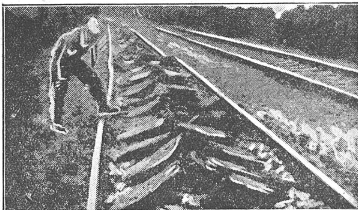
FIG. 4. — TRÂVERSES BRISÉES SOULEVÉES PAR LA MACHINE
