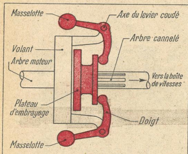
FIG. 9. — SCHÉMA D'UN EMBRAYAGE CENTRIFUGE
