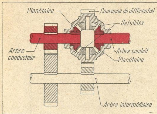
FIG. 13. — SCHÉMA DU FONCTIONNEMENT D'UN CHANGEMENT DE VITESSE À DIFFÉRENTIEL
