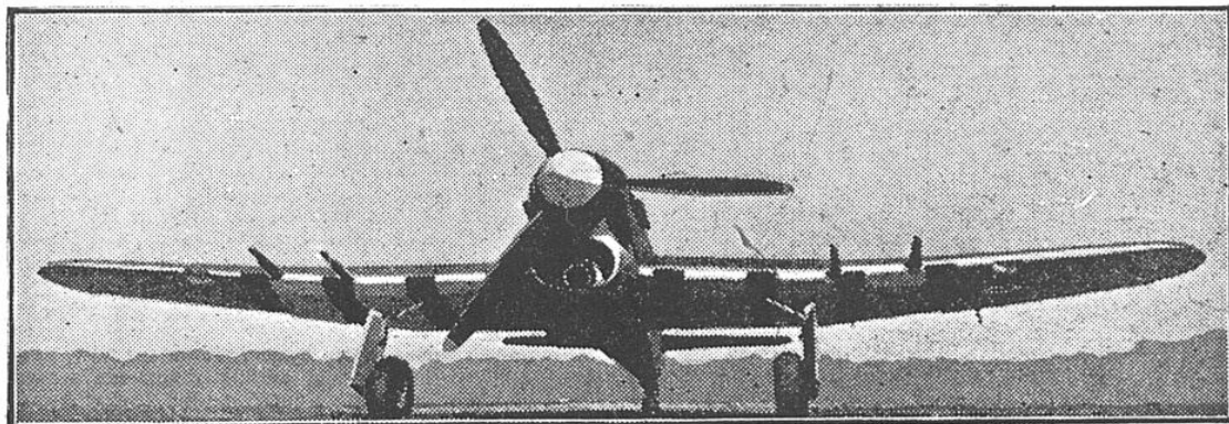
FIG. 7. — LE MONOPLANE DE CHASSE HAWKER « TYPHOON », ARMÉ DE QUATRE CANONS HISPANO DE 20 MM EST ÉQUIPÉ D'UN GRAND RADIATEUR A TUYÈRES DISPOSÉ SOUS LE MOTEUR
